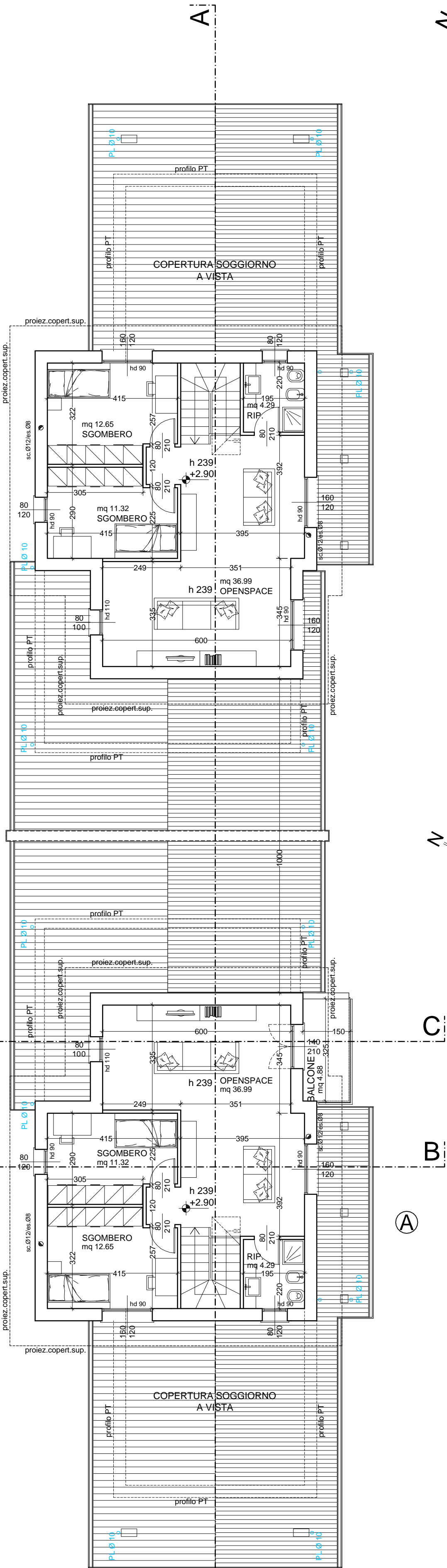
PIANO PRIMO / SOTTOTETTO AGIBILE NON ABITABILE Sc 1:100
